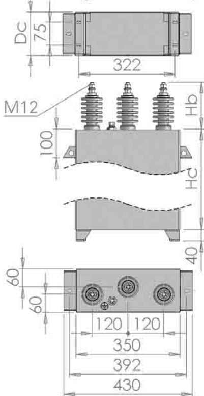
Drawing No./Rozměr. výkr. 3
