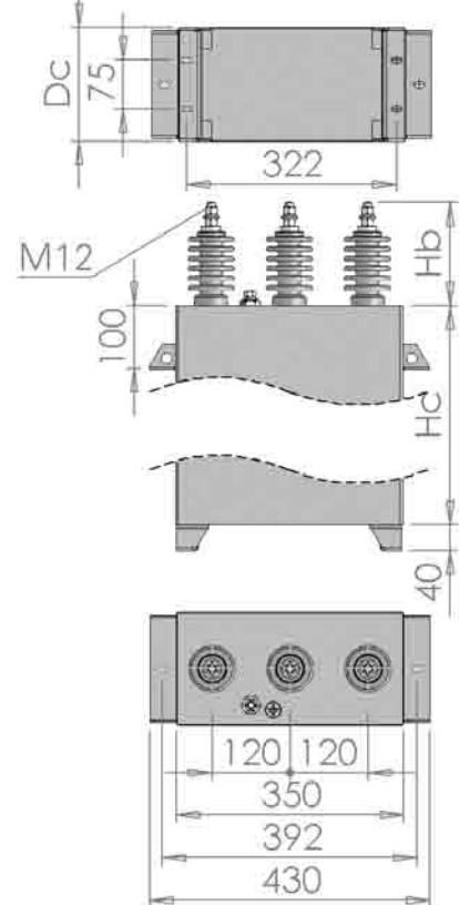
Drawing No./Rozměr. výkr. 2
