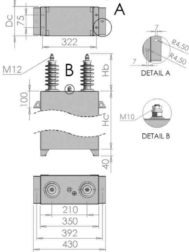
Drawing No./Rozměr. výkr. 3
