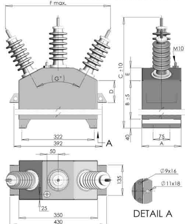
Drawing No./Rozměr. výkr. 4
